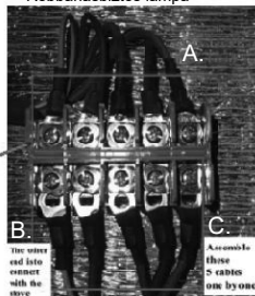
A fűtőtest kábelcsatlakozói
