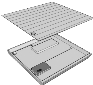
porvédő lemez
